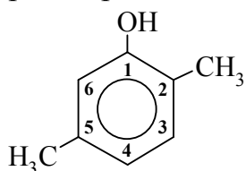
2,5-диметилфенол
