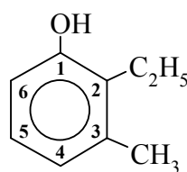
3-метил-2-этилфенол
