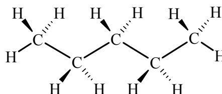
n-Пентан
